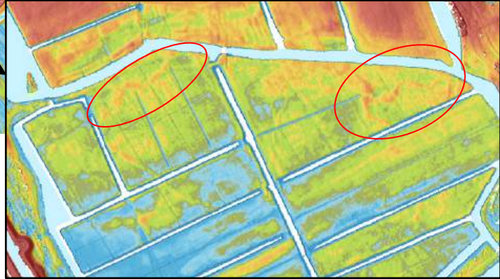
1.3 – Hoogtekaart van het Polderpark Cronesteyn en uitsnede van het park. Hoe blauwer de kleur, hoe lager gelegen het gebied. Hoe warmer (geel – rood) hoe hoger gelegen het gebied. Opvallend is dat binnen de relatief laag gelegen delen (groen gekleurd) kronkelende vormen aanwezig zijn, die hoger liggen (geel/ oranje gekleurd). Deze gebieden zijn in de uitsnede met een rood ovaal omcirkeld. Dit zijn vermoedelijke kreekruigten van uitlopers van de Holocene krekken in het gebied (Bron: AHN4)
